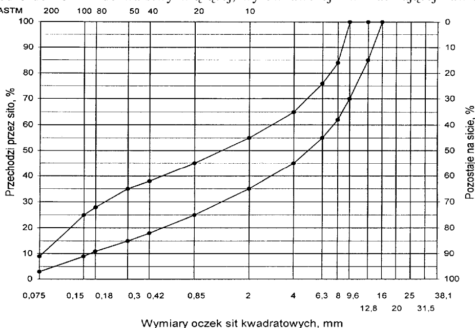
Rys. 10. Krzywe graniczne uziarnienia mieszanki mineralnej BA od 0 do 12,8 mm do warstwy wiążącej, wyrównawczej
