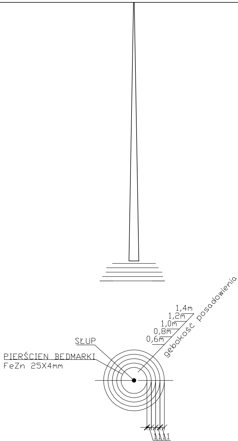
schemat posadowienia uziomów otokowych słupów oświetleniowych
