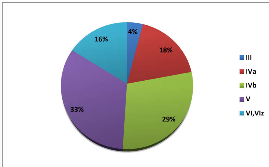
Wykres 1. Klasy bonitacyjne gleb w gminie Somianka
