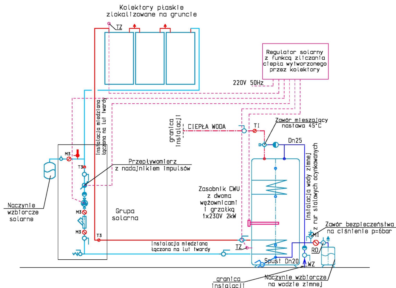
Schemat poglądowy instalacji solarnej - rysunek 1
